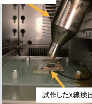
X線発生装置による 照射試験の様子
