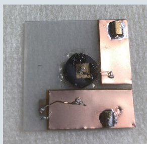
ペロブスカイトX線検出 素子試作品（MaPbI3）
