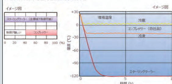
FPSCの特長：厳密な温度制御に適する
