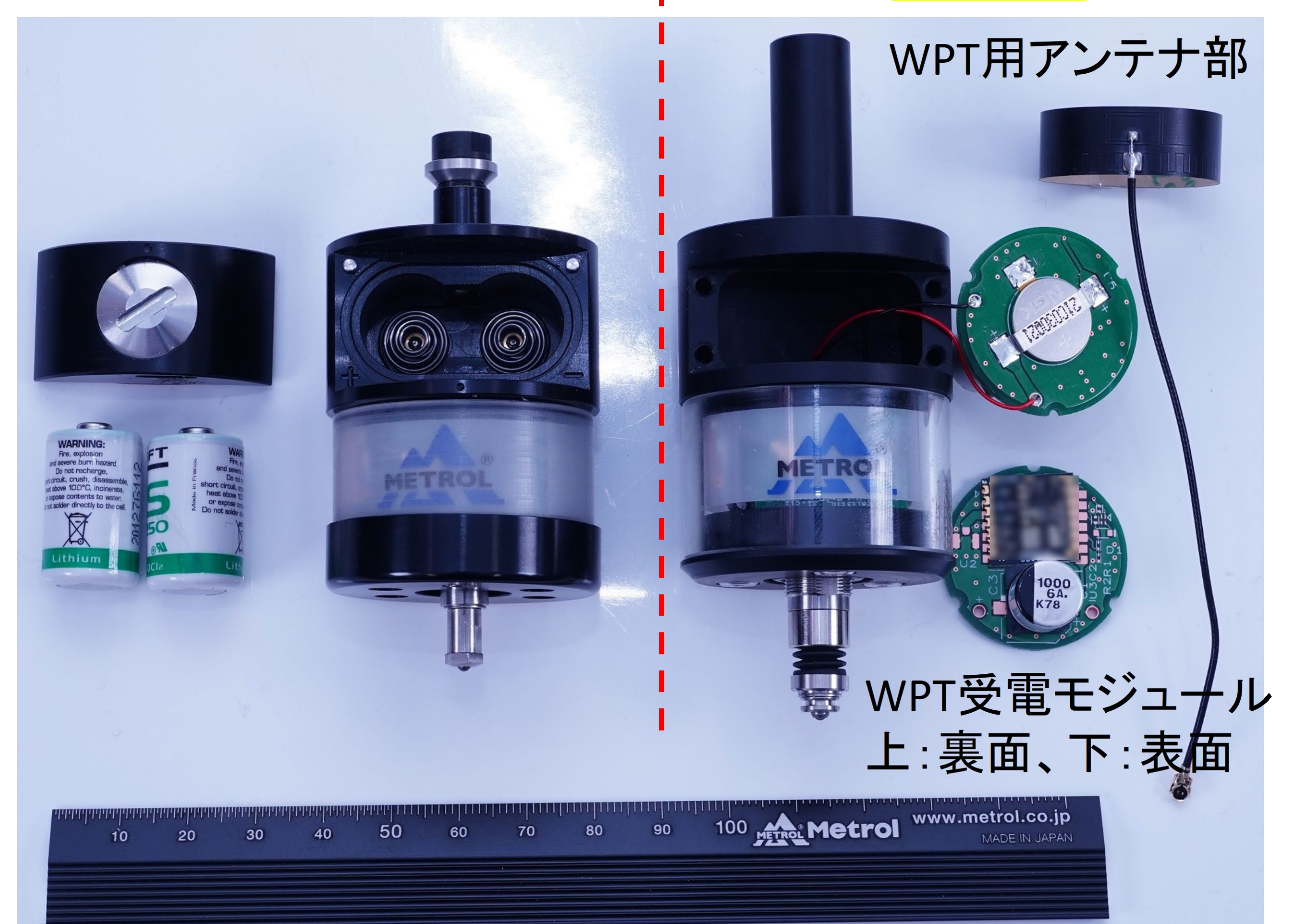
図4 現行品と開発中(WPT搭載)のタッチプローブ
