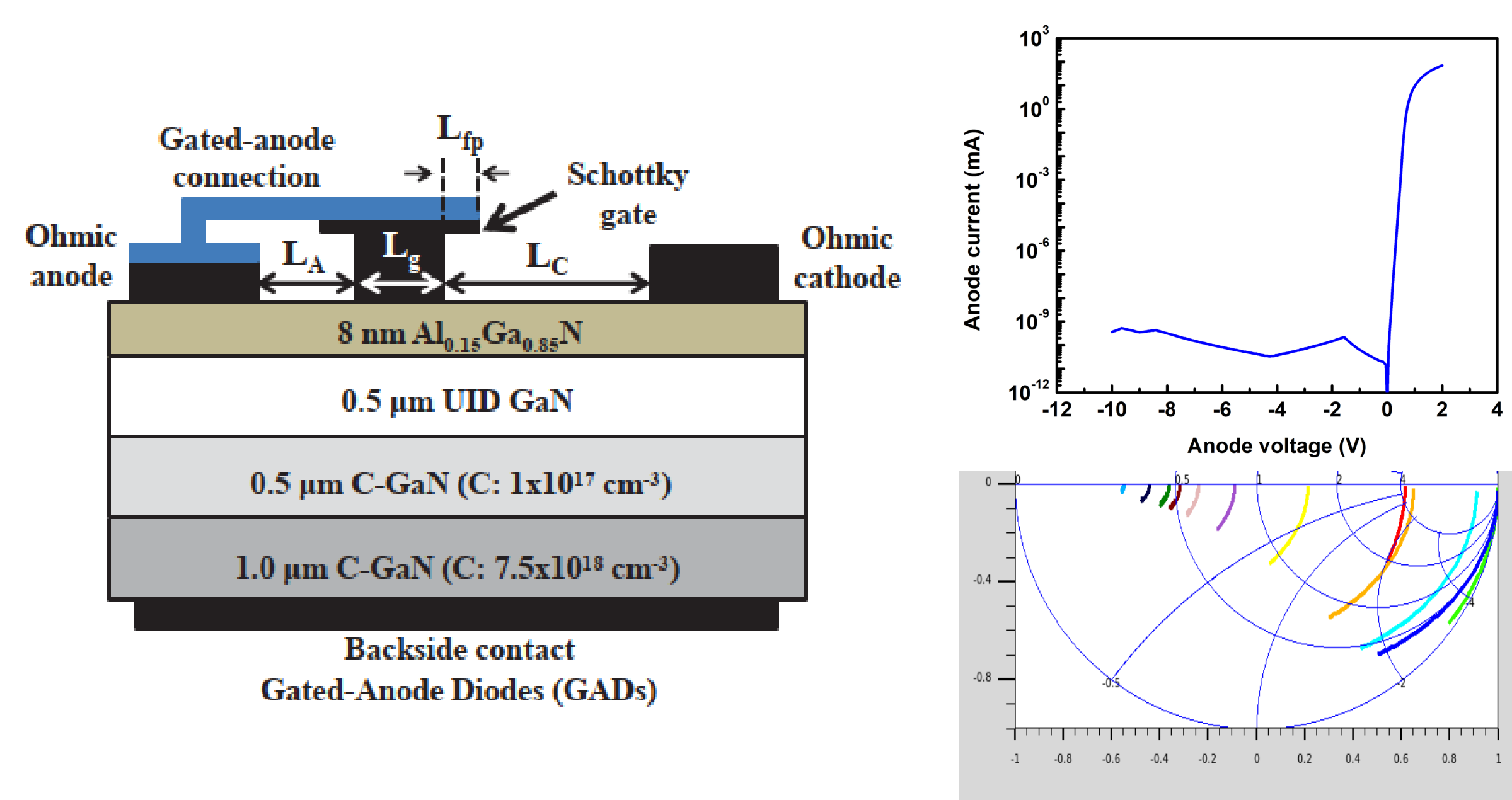
図2 ミリ波動作を検討しているGaN半導体を用いた受電整流素子とその特性予測
