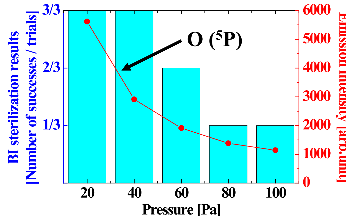
BIの滅菌結果と五重項酸素原子の発光強度の圧力変化
