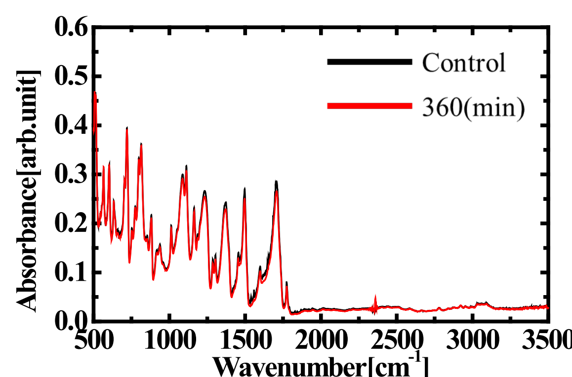
酸素プラズマ照射前後のポリイミドフィルムのIRスペクトル
